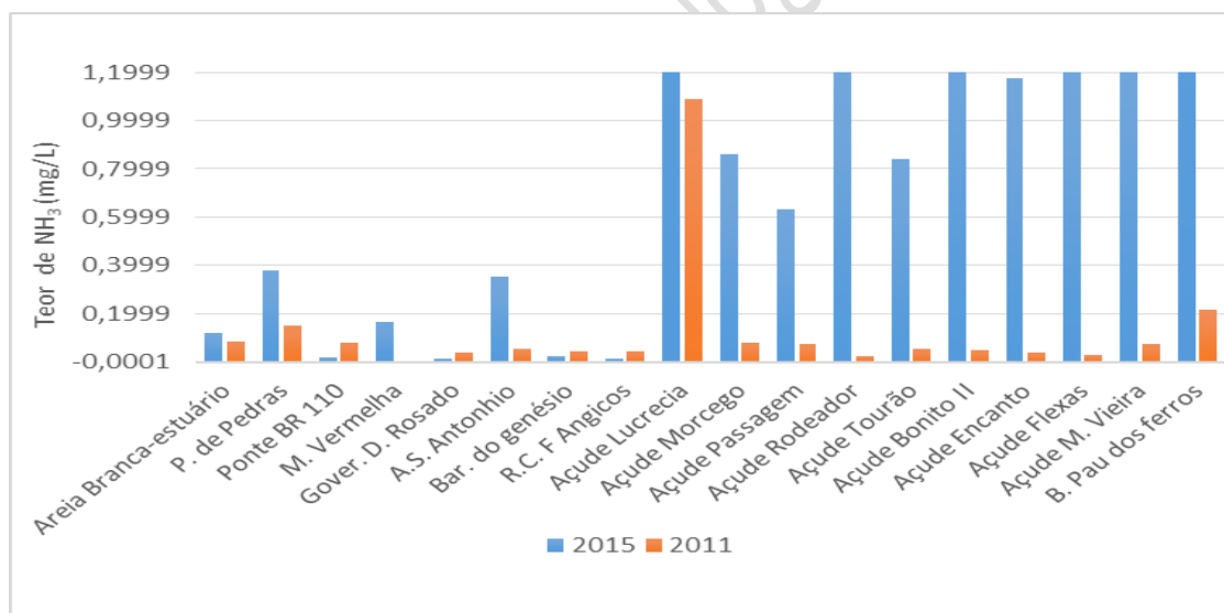
Gráfico 4: Teores de NH_3 nos 18 pontos analisados.
