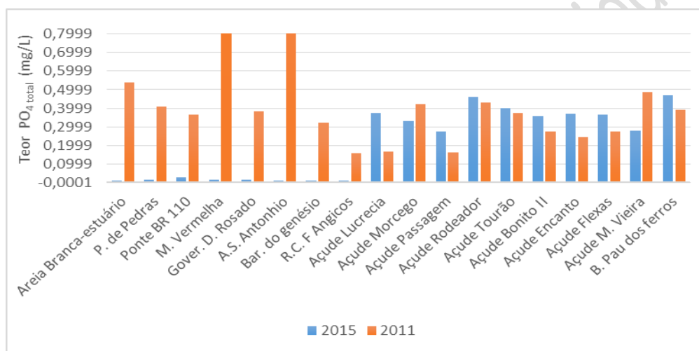
Gráfico 2: Teores de PO 4 total nos 18 pontos analisados.
