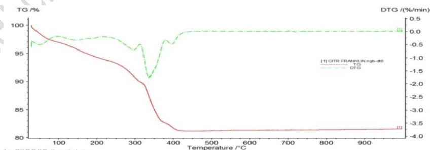
Figura 2. Curva Termogravimétrica do Citrato de Níquel
