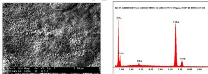
Figura 6 : (a) Imagem micrográfica e (b) espectro da superfície do aço em HCl 1 M na presença do extrato (1000 ppm) após o tempo de imersão de 24
