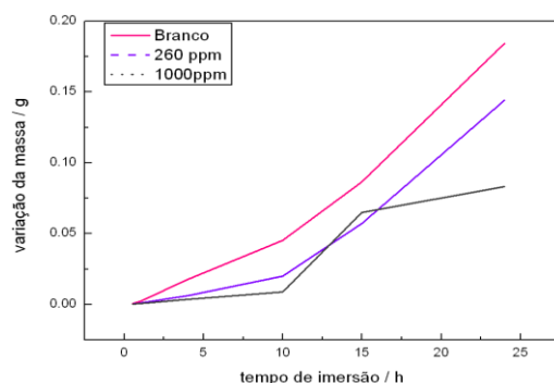
Gráfico1: Variação da perda de massa do aço carbonado em HCl 1M com o tempo de imersão.
