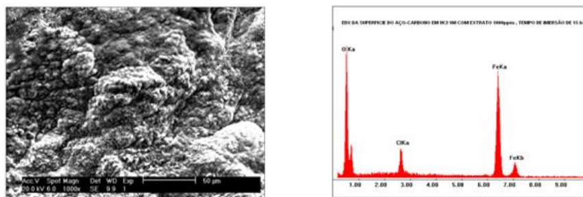
Figura 5 : (a) Imagem micrográfica e (b) espectro da superfície do aço em HCl 1 M na presença do extrato (260 ppm) após o tempo de imersão de 24 h
